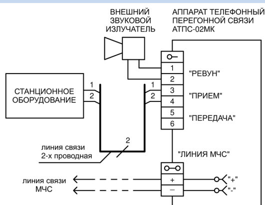
К 2-Х ПРОВОДНОЙ ЛИНИИ СВЯЗИ
